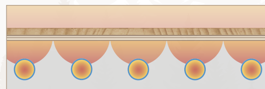
WÄRMEVERTEILUNG BEI FUßBODENHEIZUNG
